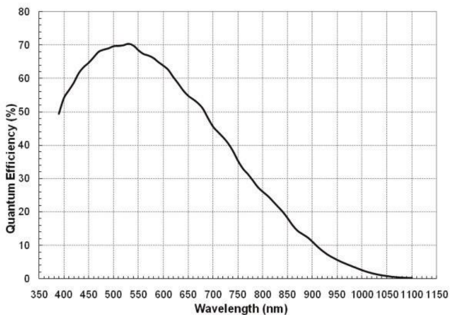
图 1 光谱响应图
