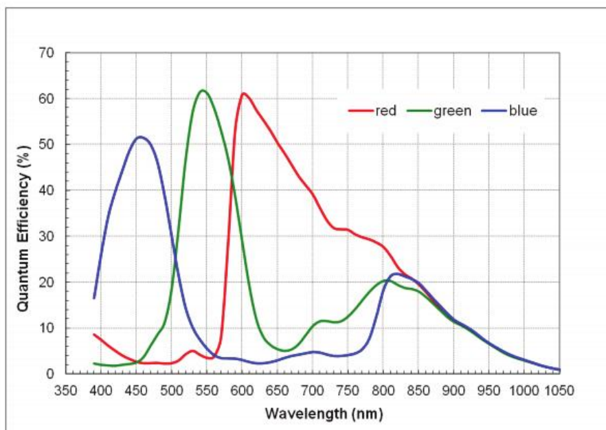
图 1 光谱响应图
