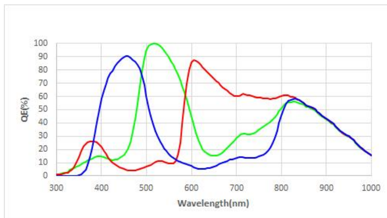
图 1 光谱响应图
