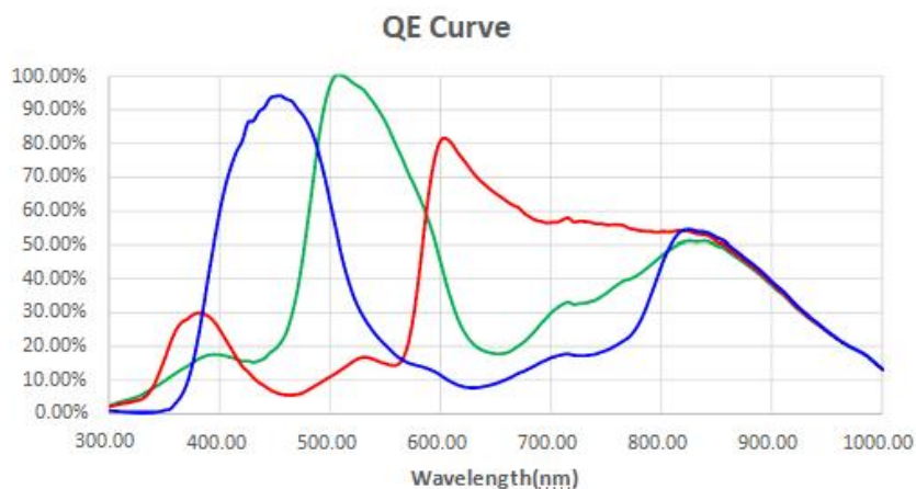
图 1 光谱响应图
