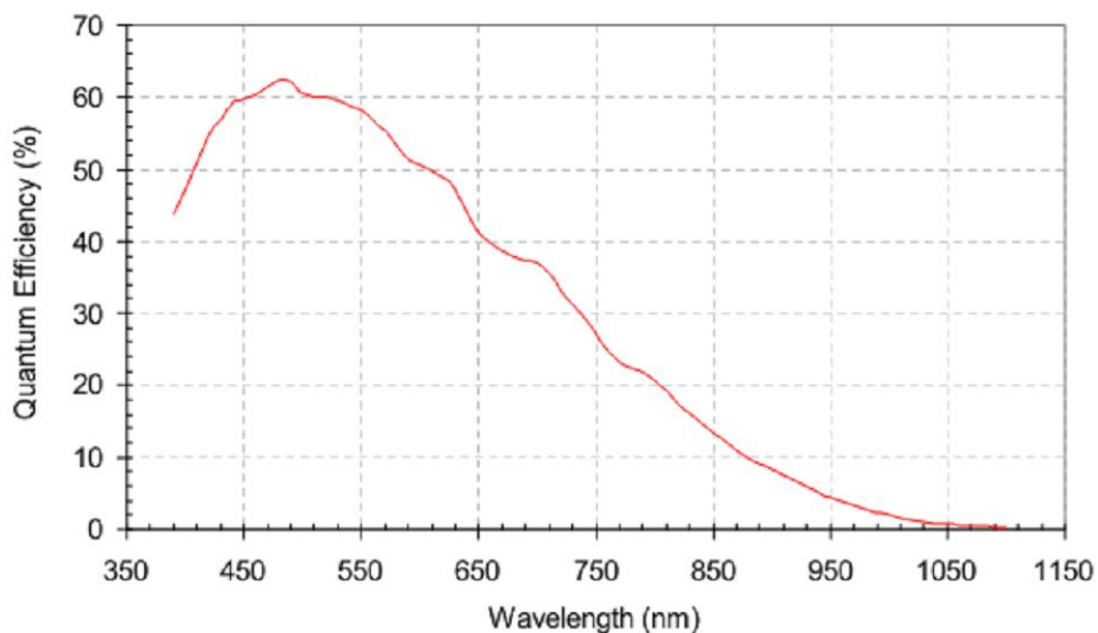
图 1 光谱响应图
